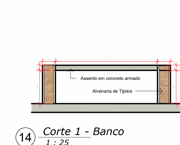
14 Corte 1 - Banco 1 : 25
