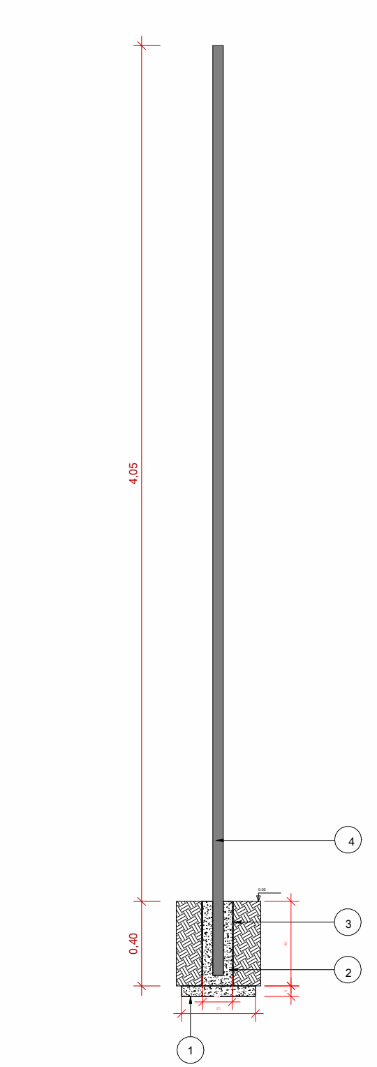
Det. Fixação Alamedado 1 : 25
