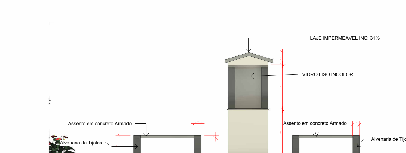
11 Vista 1 Obelisco e Bancos 1 : 50
