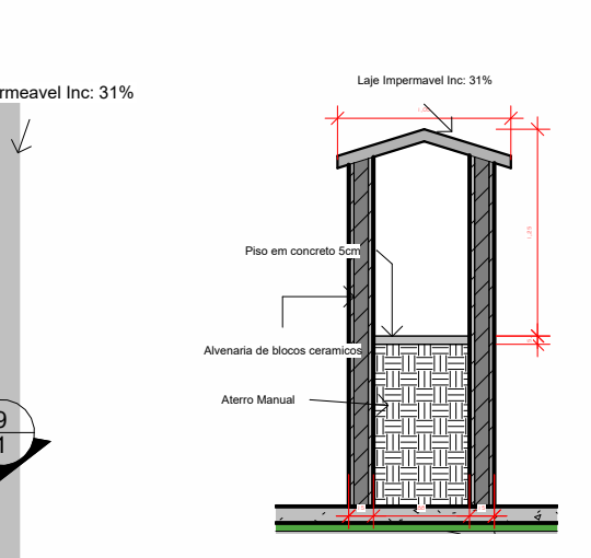
9 Corte 1 - Obelisco 1 : 50
