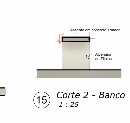
15 Corte 2 - Banco 1 : 25
