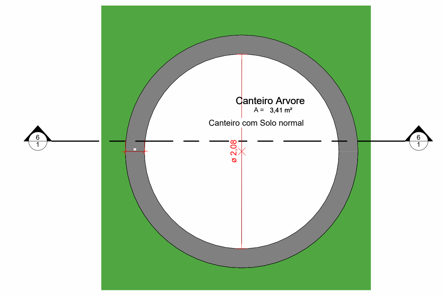
5 DET. MURETA DAS ÁRVORES 1 : 25
