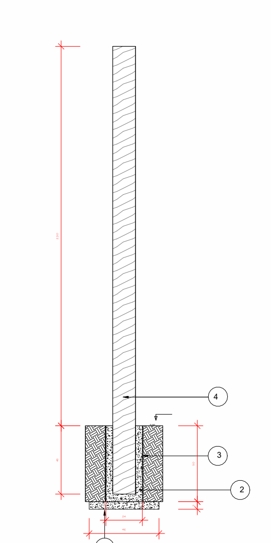
Det. Fixação Pergolado 1 : 25
