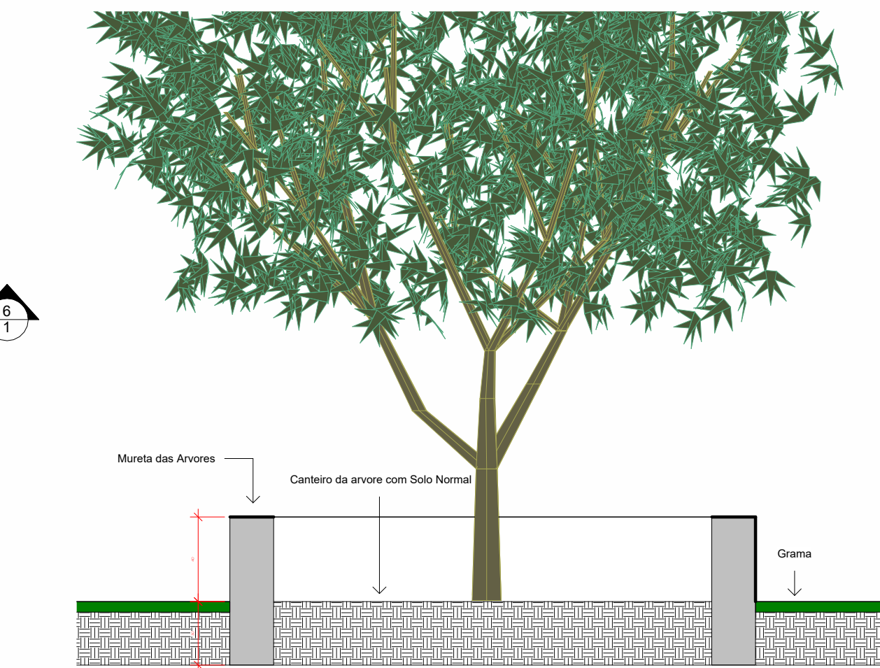
6 Corte Mureta Arvore 1 : 25
