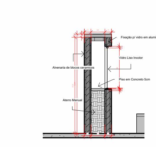
10 Corte 2 - Obelisco 1 : 50
